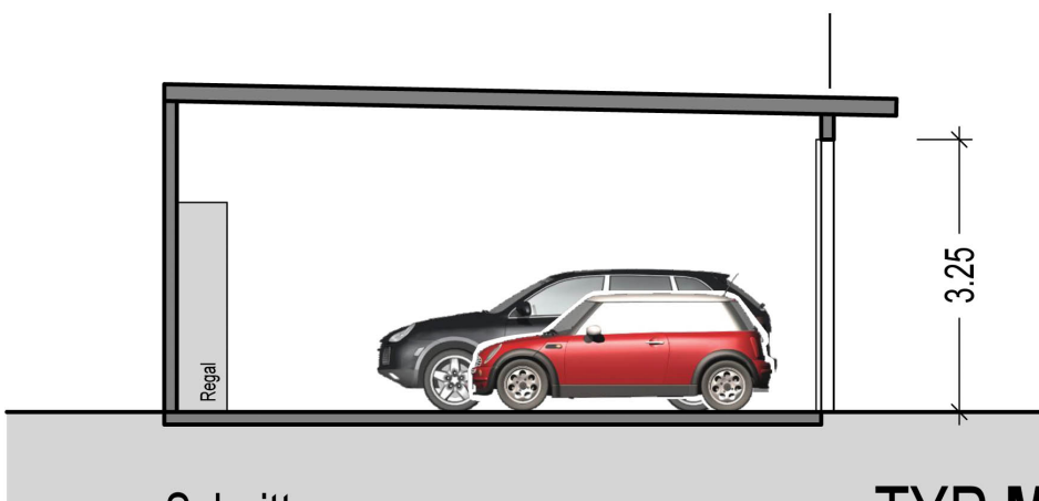
Schnitt
